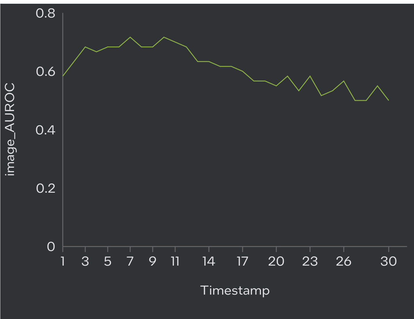
image_AUROC
