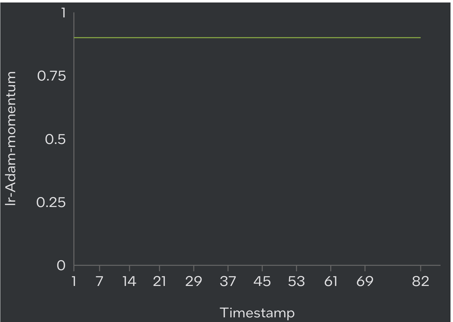
lr-Adam-momentum
